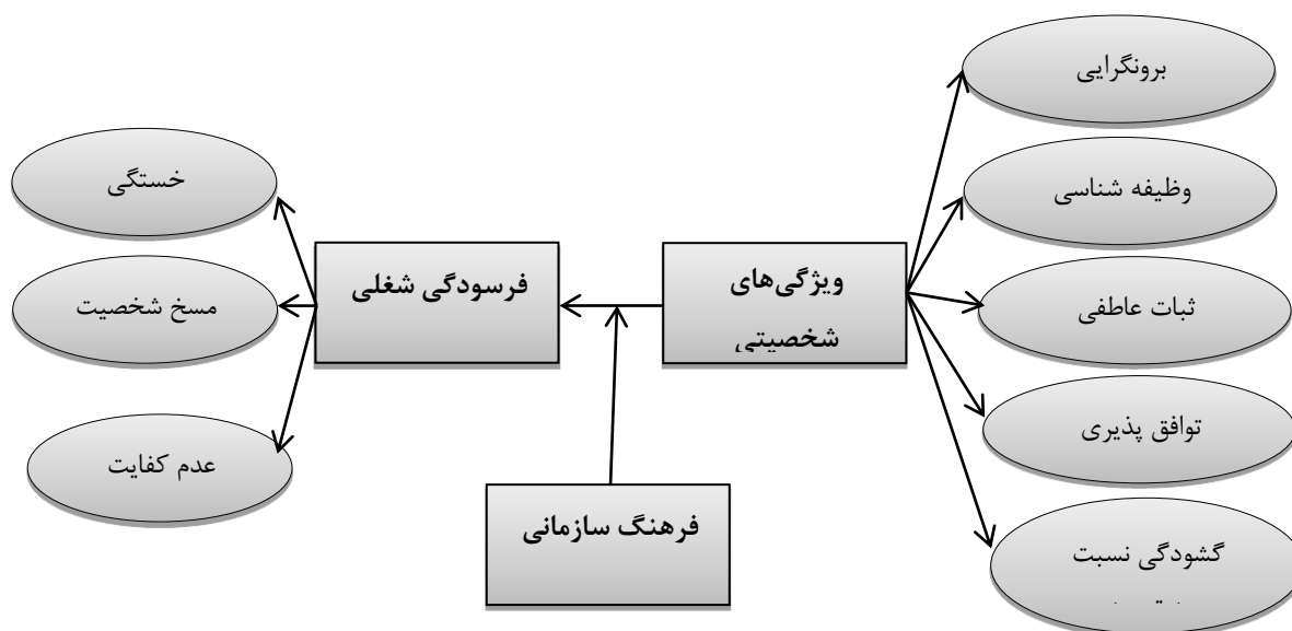
شکل ۱- مدل تحقیق (آزاده، ۱۳۹۴)
