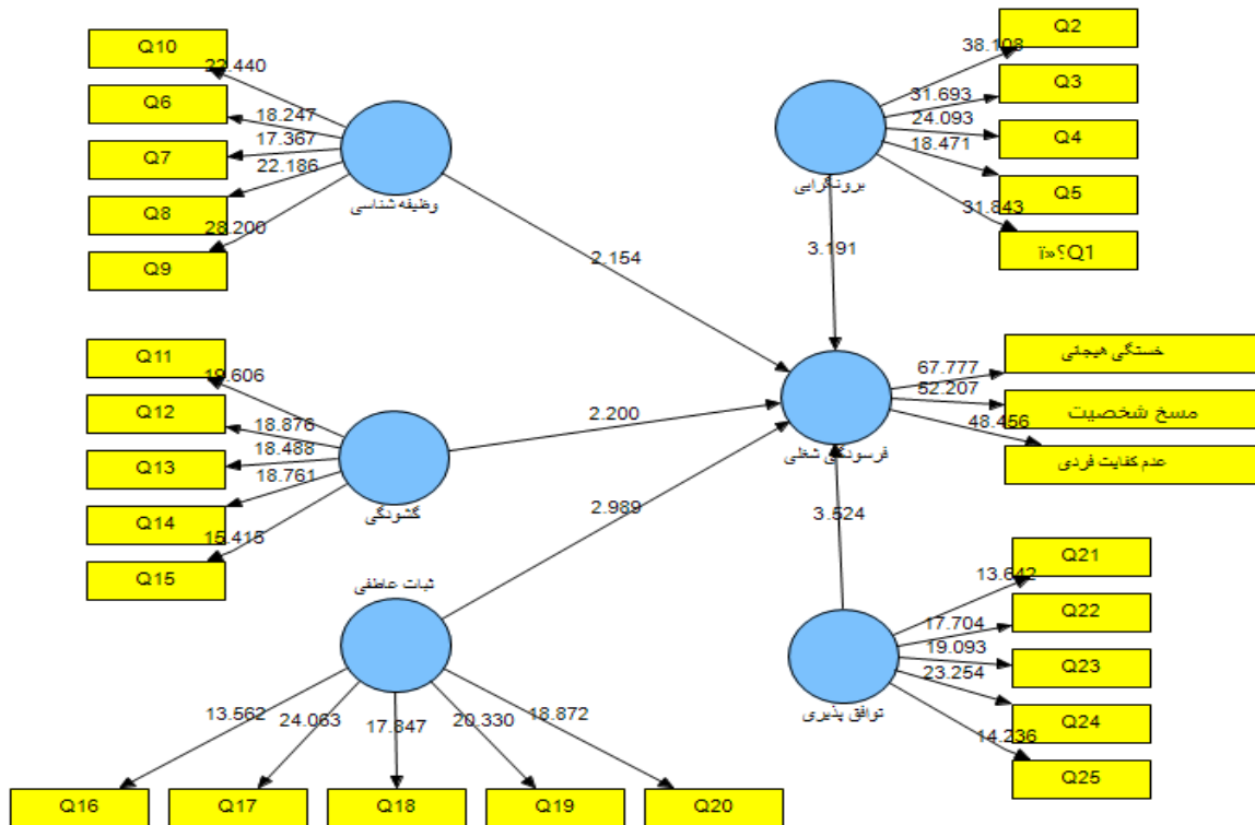
شکل ۵- خروجی نرم افزار- ضرایب t مربوط به فرضیات پژوهش
