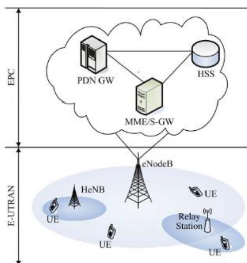
شکل ۷ ساختار معماری LTE.
